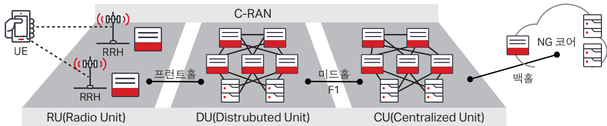
그림 2. 5G NR RAN 아키텍처
