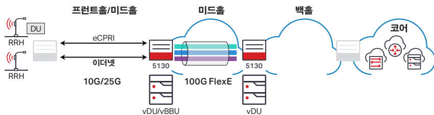
그림 1. Cloud-RAN 네트워크 애플리케이션
