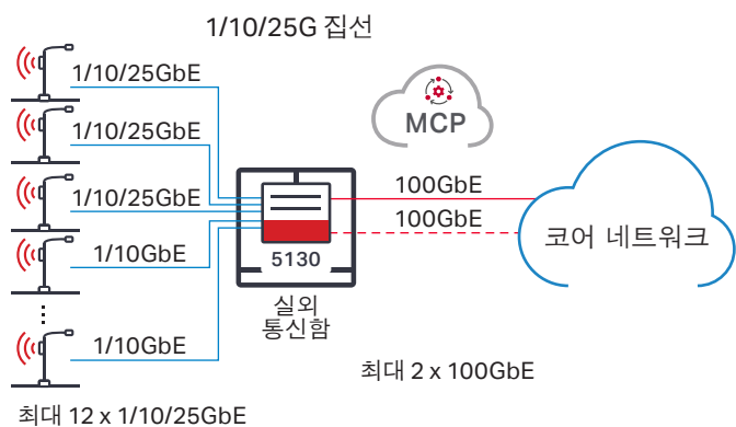
그림 3. 5130 라우터 옥외 서비스 및 집선
