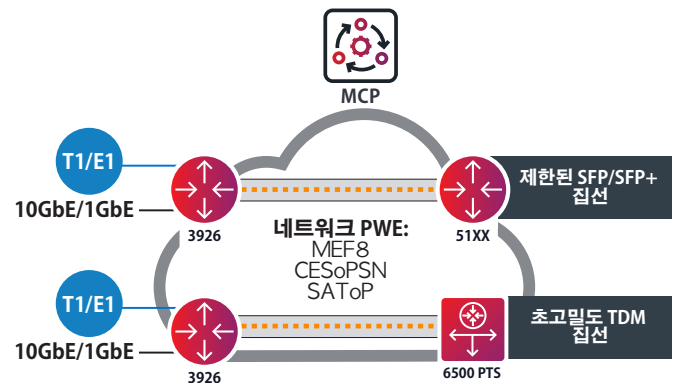
그림 6. Ciena 3926 플랫폼
